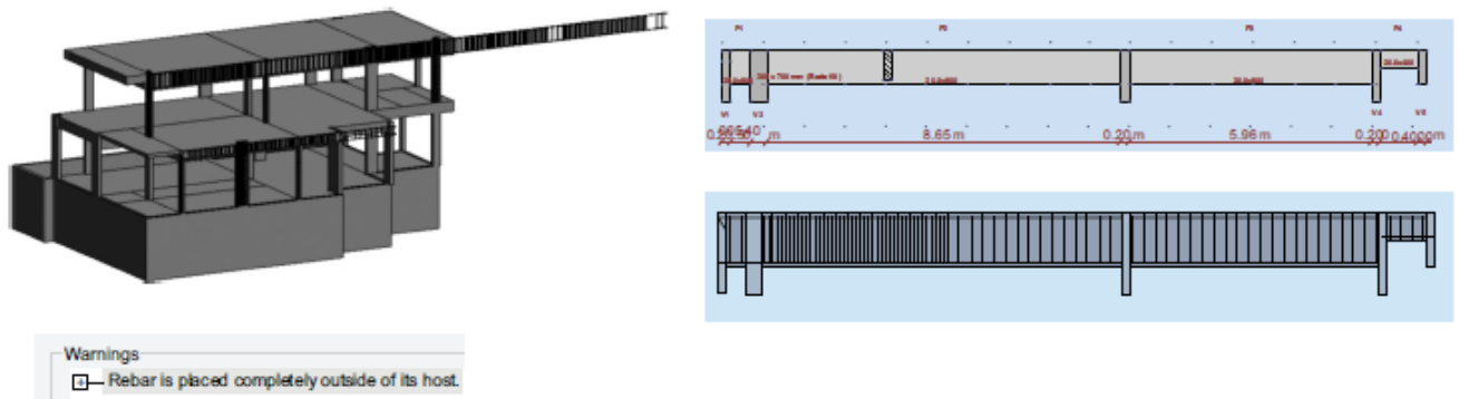
Рис. 4.10. Помилка при передачі в Revit через визначення балки як безперервної на всіх прольотах у Robot
