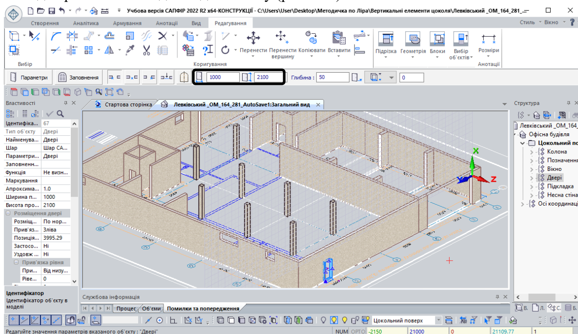
Рис.8.11 Призначення дверного прорізу
