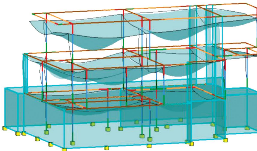
Рис. 4.22. Деформації плити
