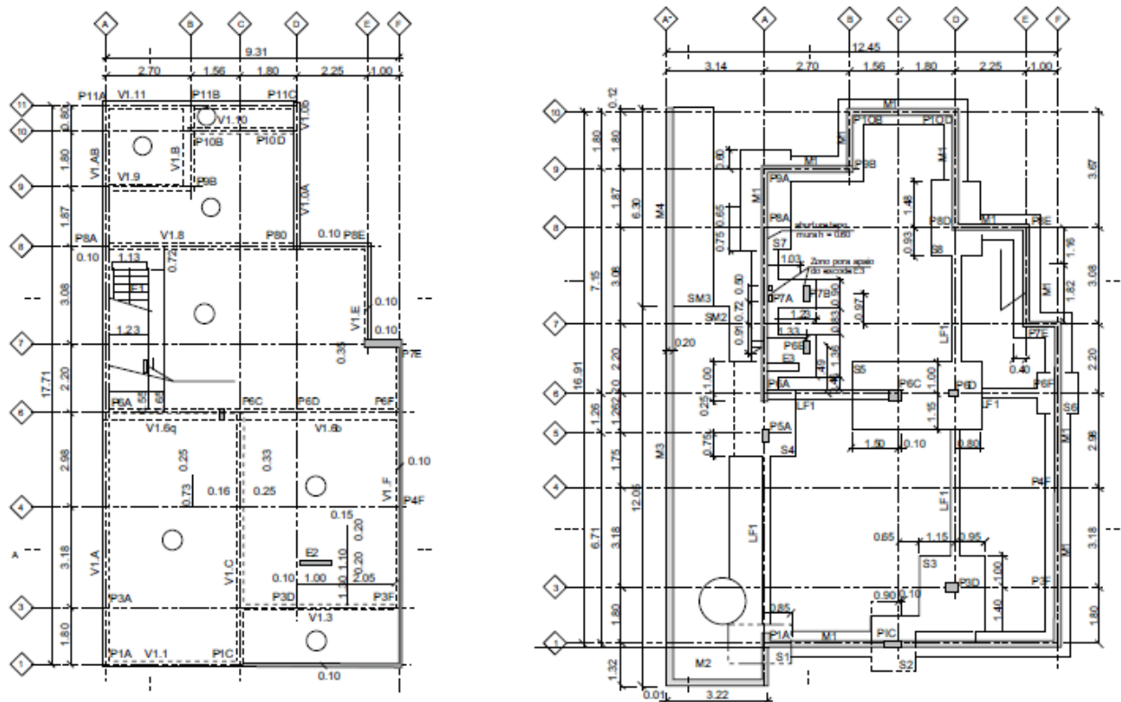
Рис. 3.2. Технічні креслення конструктивного проєкту
