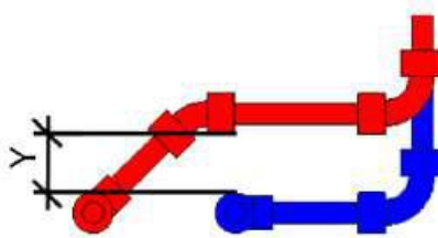
Рис 4.124 - Відстань у світлі [Y]
