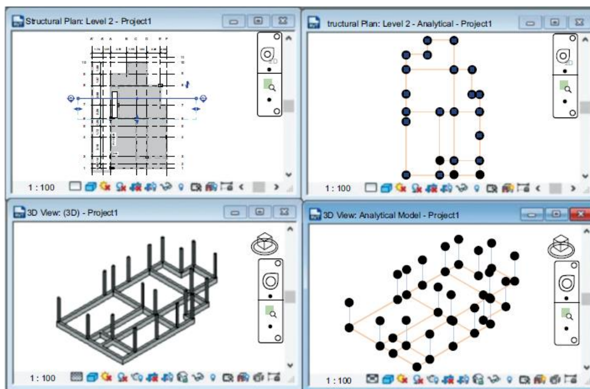
Рис. 3.11. Порівняльне представлення геометричної та аналітичної моделей
