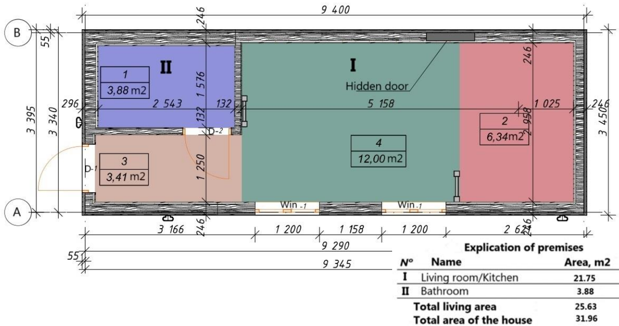
Рисунок 2.4 – План приміщень
