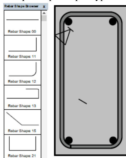
Рис. 4.12. Інтерфейси розширень арматури Revit: балка
